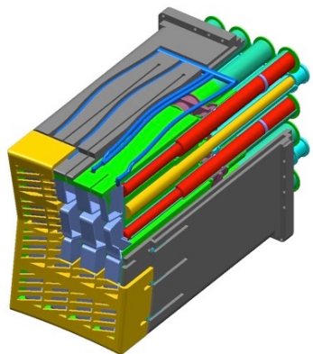
ICRH antenna
